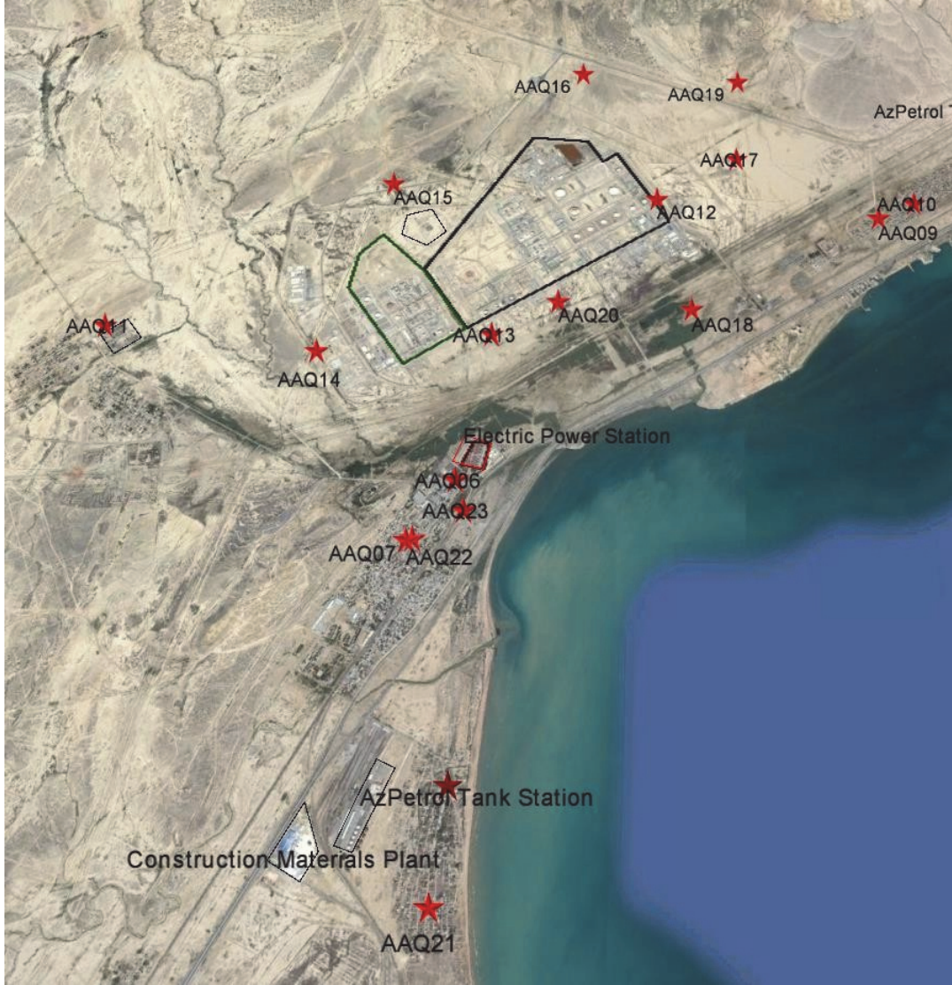
Şəkil 3.1: Nümunəgötürmə yerləri – Səngəçal Terminali
